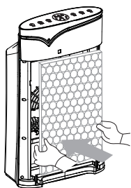
7 裝入面板，先放入頂 部V形軌道，版面底 部往內推，底部磁石 自動合上
